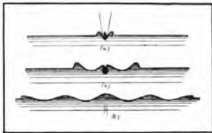
Fig. 31 - Moto ondulatorio alla superficie dell'acqua.
