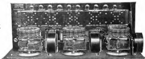
Chassis del FRESHMAN MULTIPLE visto dall'alto.
