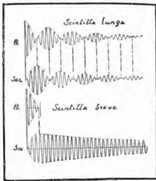
Fig. 47. - Paragone fra il sistema a scintilla normale (lunga) e scintilla frazionata (breve).
