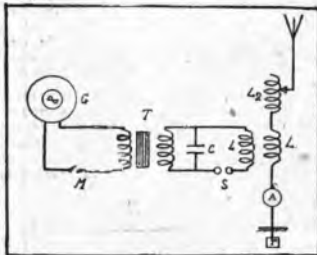
Fig. 46. - Costituzione schematica di un trasmettitore a scintilla.
