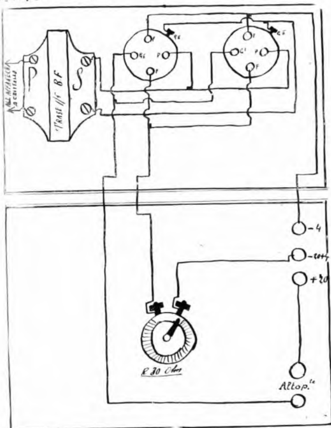
Schema di montaggio amplificatore bithodico (Abb. O. Gelmi).
