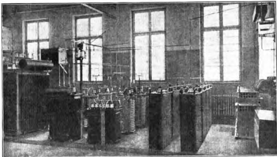
Complesso raddrizzatore - livellatore per la tensione anodica delle valvole generatrici
