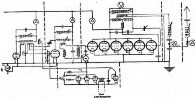
Schema elettrico circuito generatore - modulatore - amplificatore
