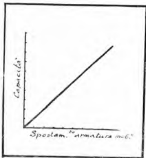
Fig. 145 - Diagramma caratteristico condensatore a variazione lineare di capacità.
