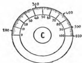
Fig. 150. Distribuzione delle varie stazioni su un quadrante del condensatore a variazione lineare di frequenza.
