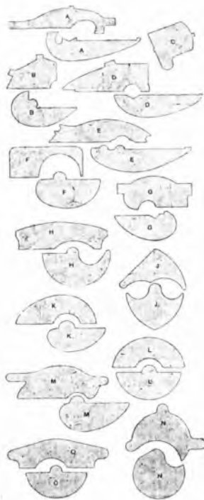
Fig. 151. Varii profili di lamette per condensatori variabili: A, B, D, E, F, lineari con la frequenza; C, G, H, J, K, M, N, O, quadrate; L, lineari
