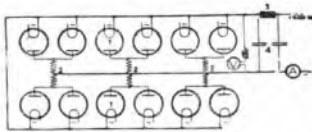
Schema elettrico circuito raddrizzatore
