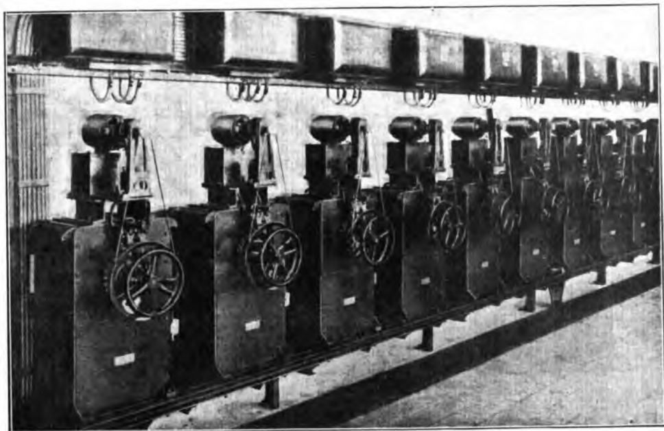
Comandi automatici azionati da servomotori elettrici
