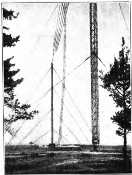
Veduta generale dell'impianto a base di uno degli alberi d'antenna con contrappeso tenditore dell'aereo.
