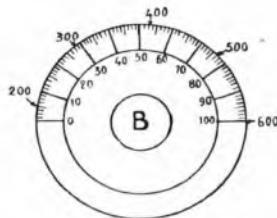
Fig. 149 - Distribuzione delle varie stazioni su un quadrante di condensatore a variazione quadratica.
