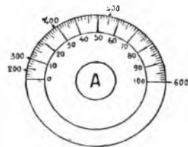
Fig. 148 - Distribuzione delle varie stazioni su un quadrante di condensatore a variazione lineare di capacità.
