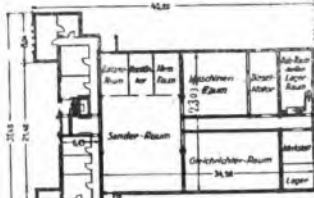
Pianta generale edificio del trasmettitore.
