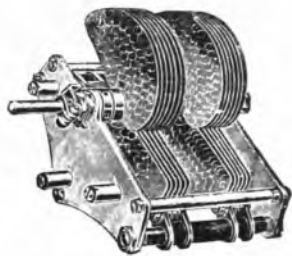
Fig. 153. Condensatore doppio a variazione quadrata.
