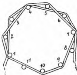
Fig. 165. Sistema d'avvolgimento delle bobine a gabbione
