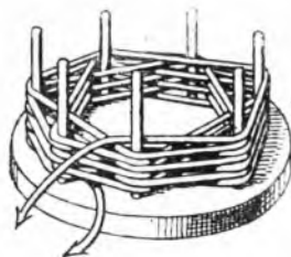
Fig. 166. Bobina a gabbione in costruzione
