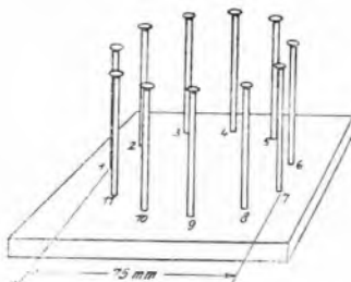
Fig. 164. Scheletro per la costruzione di bobine a gabbione
