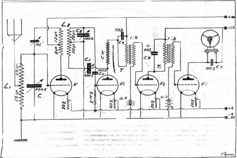
Schema del Radiorecettore a 4 valvole
