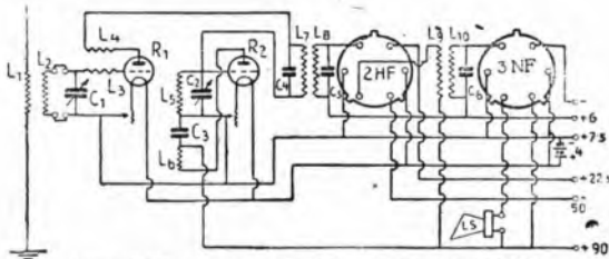
Apparecchio Ultradina con una Bivalvola e una Trivalvola "LOEWE".
