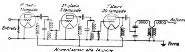
Fig. 5. - Schema semplificato dell'amplificatore ad alta frequenza.
