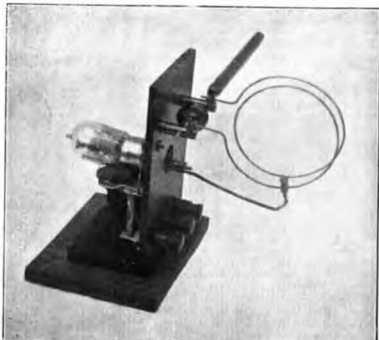
Oscillatore autodina sensibile alle onde di lunghezza 1-5 metri
