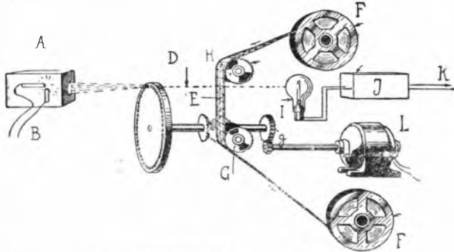
Figura 1 - Schema di principio del trasmettitore telecinematografico.
