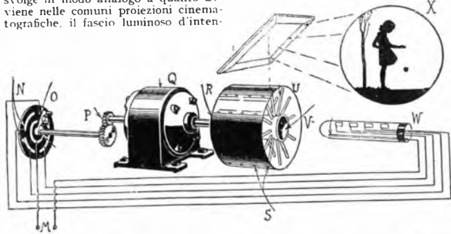
Figura 2 - Schema di principio del ricevitore telecinematografico.
