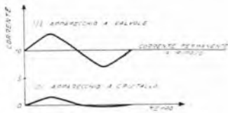
Fig. 3 CURVE DI CORRENTE NEL RICEVITORE TELEFONICO COLLEGATO LORE IN UNO DEI DUE TIPI
