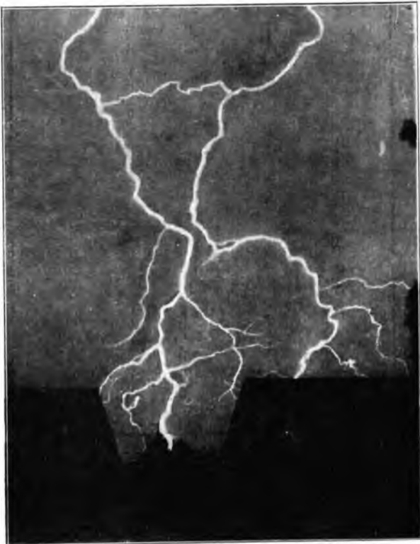
Un fulmine artificiale. Per lo studio dei fenomeni elettrometeorici, in un grande laboratorio americano si sono riprodotti dei fulmini artificiali lunghi quasi otto metri
