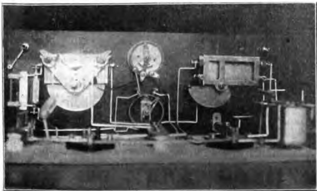
L'apparecchio montato
