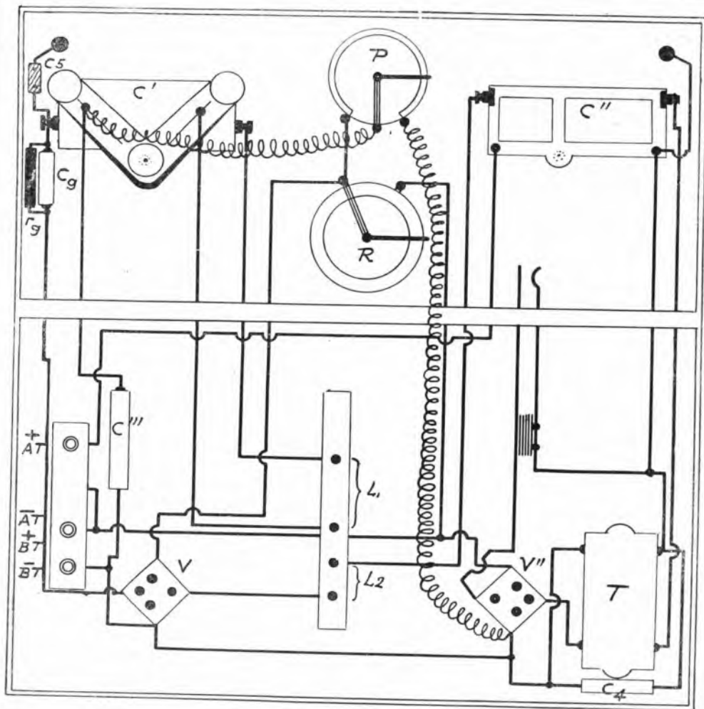
Schema di montaggio.
