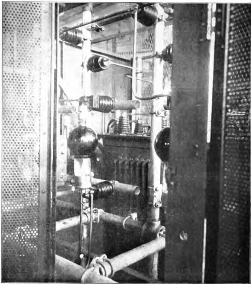
Rettificatore a vapore di mercurio (hot-cathode) della R.C.A. per la STAZIONE NAZIONALE DI ROMA DA 50 KW.
