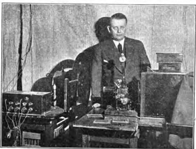
Il Radiotecnico Dénis Mihaly innanzi al suo apparecchio per mezzo del quale si può ricevere in casa la televisione
