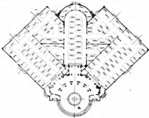
La pianta del padiglione Elettrotecnico-Radio
