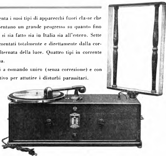
Apparecchio tipo « 700 E » in alternata sette valvole (fra cui due schermate) con combinazione elettro-grammofonica in cassetta completamente in fusione alluminio funzionante da schermo.
