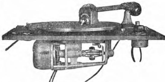
ELECTROVOX Phonomotor e Phonovox montati su tavola formante piano superiore del fonografo con ogni altro accessorio L. 1200.
