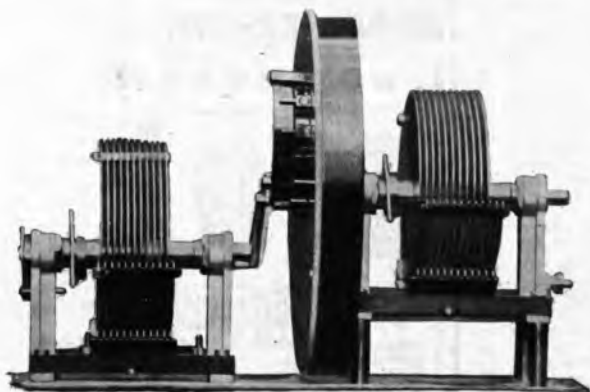
Selettore ad Unico Comando R. R. R. Tipo Simplex
