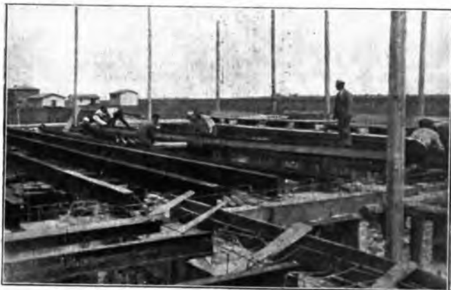
Fig. 1 - Edificio del trasmettitore - Copertura della grande Sala-macchine
