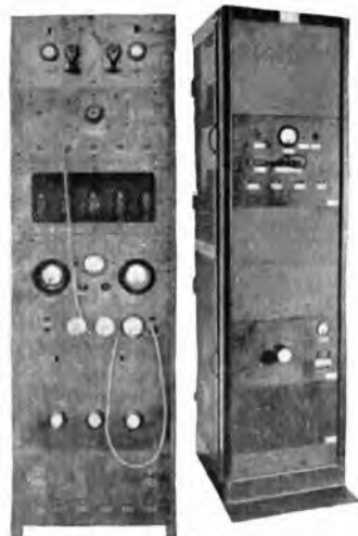
Tipi di amplificatori usati nei film sonori
