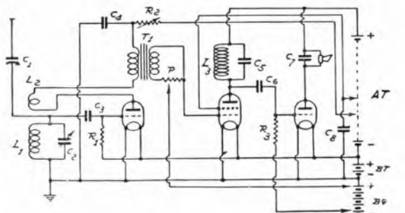
Fig. 2. Ricevitore a tre valvole C_1 compensatore 0.0001 mfd; C_2 condensatore variabile (vedi testo); C_3 = 0.0001 mfd; C_4 = 1 mfd; C_5 = 0.07 mfd; C_6 = 0.0005 mfd; C_7 = 0.002 mfd; C_8 = 1 mfd; R_1 = 3 megohm; R_2 = 50.000 ohm; R_3 = 8 megohm; R_4 = 200.000 ohm; L_1 induttanza di sintonia; L_2 bobina di reazione
