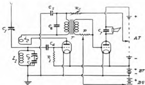
Fig. 3 - Ricevitore a due valvole C_1 compensatore 0.0005 mfd; C_2 compensatore 0.0001 mfd; C_3 condensatore variabile di 0.0005 mfd; C_4 = 0.0001 mfd; C_5 = 1 mfd; C_6 = 0.002 mfd; C_7 = 0.0002 mfd; C_8 = 3 megohm; R_1 = 3 megohm; R_2 = 50.000 ohm; R_3 = 200 ohm; L_1 indut. di sintonia; L_2 bobina di reaz.; T. trasform. BF/AF.
