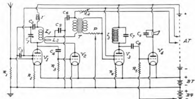
Fig. 1 - Ricevitore a quattro valvole
