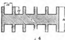
Rocchetto per l'avvolgimento della induttanza per il circuito accordato BF.
