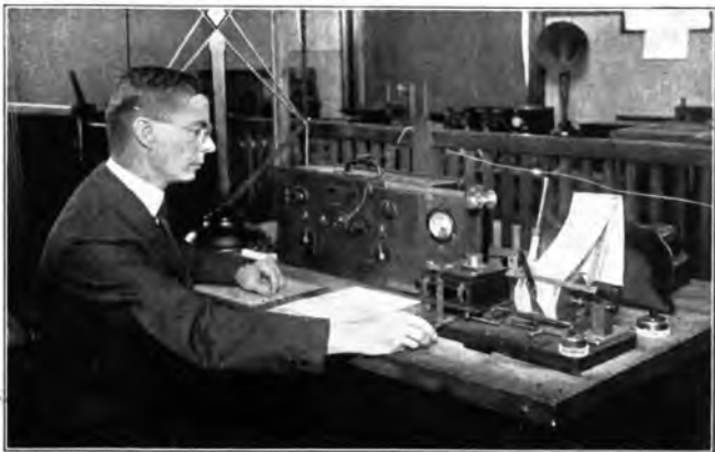
Un impianto di registrazione del «fading» nel laboratorio del Bureau of Standard a Washington, a scopo di indagine su questo fenomeno ancora non completamente conosciuto
