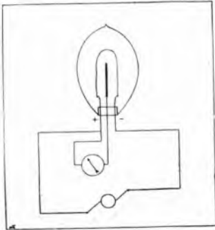
Fig. 4. — Circuito dimostrativo dell'effetto Edison.
