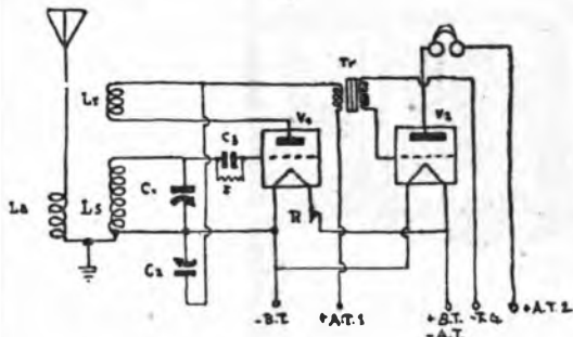
Fig. 1. - Schema teorico del ricevitore per onde corte.
