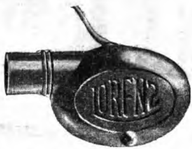
PICK UP con cordone e spina
