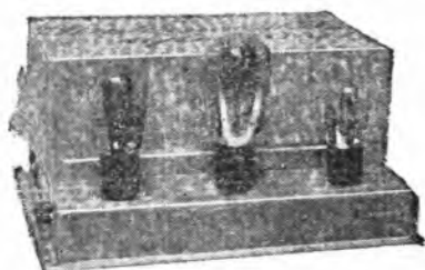
Tipo NF 30 e 30 R per una potenza modulata utile di 2,5 a 3 watt
