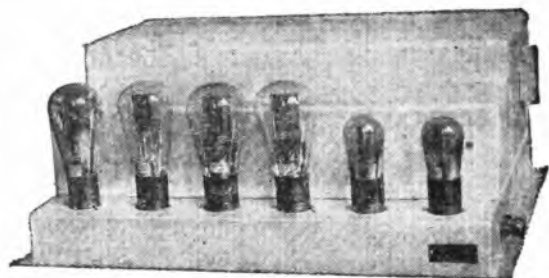
Tipo NF 50 e 50 R per una potenza modulata utile di 12 a 14 watt e Tipo NF 60 per 15 watt
