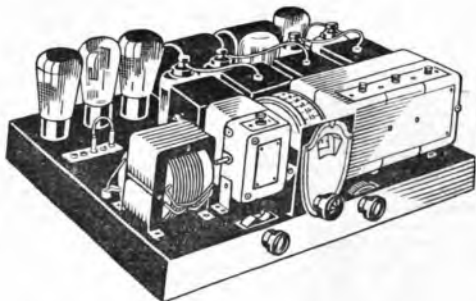
Chassis Modello R. 85, completo di nove valvole Philips, quattro schermate, potente e melodioso, adatto per qualsiasi tensione e per qualsiasi diffusore dinamico o magnetico: Lire 2150 .
