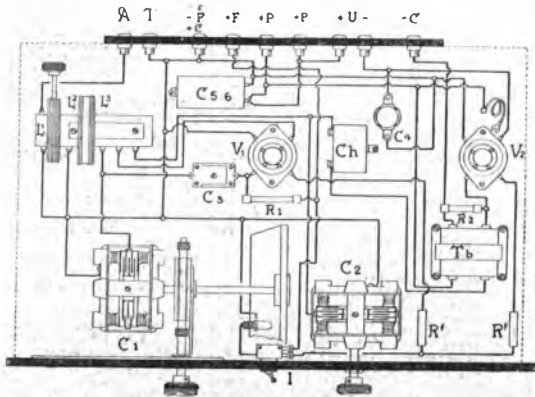
Piano costruttivo.
