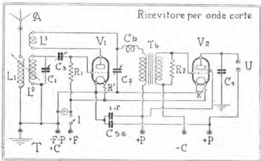
Schema elettrico.
