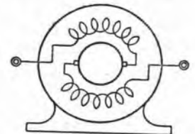
Fig. 5. - Motorino a montaggio simmetrico: gli avvolgimenti dello statore fanno da impedenza.
