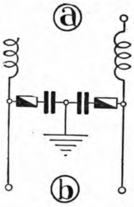
Fig. 1. - Schema del dispositivo classico per la circoscrizione dei disturbi in (b).
