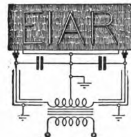
Fig. 9. - Un impianto al neon secondo le prescrizioni dell'U.R.
