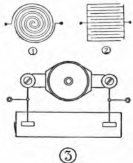
Fig. 2. - Tipi di condensatori: (1) elettrodi a spirale; (2) condensatore senza induttività; (3) coppia a impedenza nulla per tutte le frequenze.
