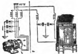
Fig. 8. - Come si circoscrivono i disturbi industriali.
