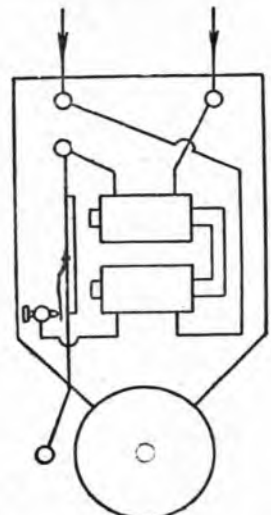
Fig. 4. - Campanello a montaggio simmetrico.
