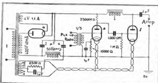
Schema dell'amplificatore.
