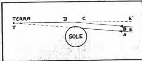
Il disegno indica la deviazione che un raggio luminoso BCDT proveniente da una stella lontana, è o raggiunge la Terra T subisce in vicinanza del Sole. La parte iniziale BC e quella DT in realtà sono diritte ed un osservatore (terrestre), ricevendo il raggio luminoso secondo DT, crede che la stella si trovi in questa direzione e quindi in E'. Mentre senza la presenza del Sole egli riceverebbe tale raggio secondo la linea TA.
