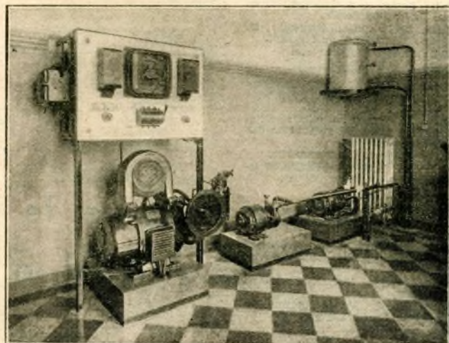
Il regolatore di tensione e le pompe per la circolazione dell'acqua.
