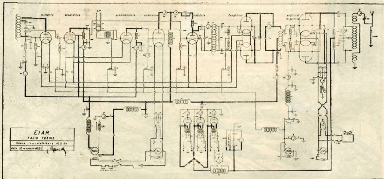
I moderni circuiti del trasmettitore.
