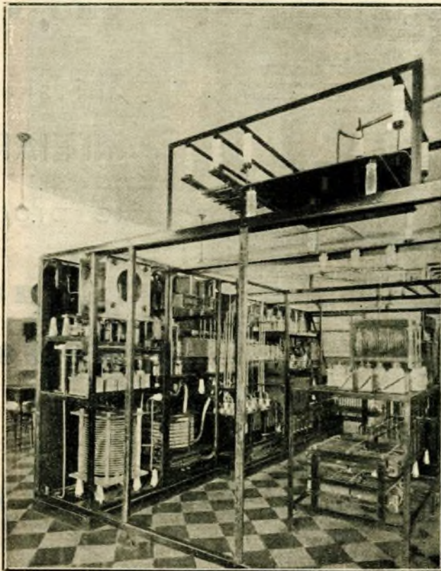
Interno del nuovo trasmettitore.
