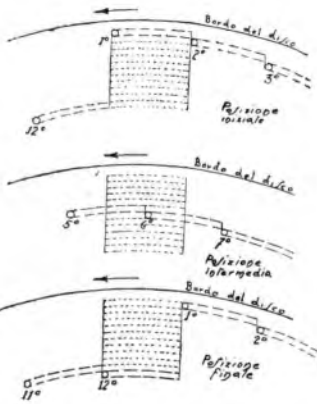
Successive posizioni dei fori in un disco analizzatore in movimento.
