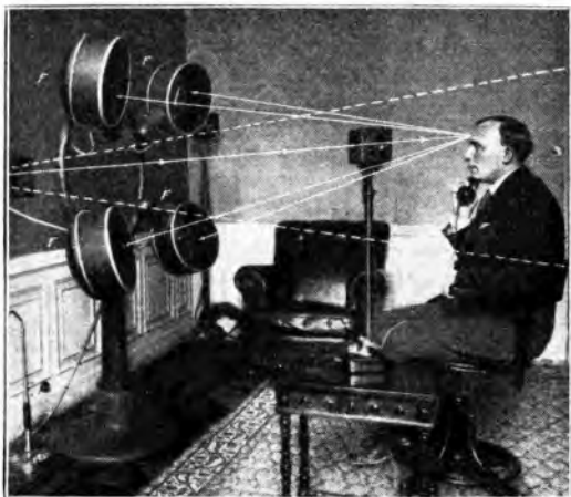
Realizzazione pratica del sistema di analisi diretta ad a raggio mobile. F fotocelle
