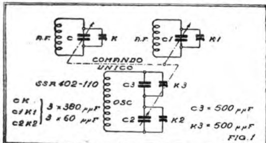
Il comando unico di una super effettuato con un condensatore triplo a tre elementi uguali.
