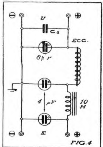
Esempio tipico di filtro provvisto di prefiltra e di condensatore supplementare.
