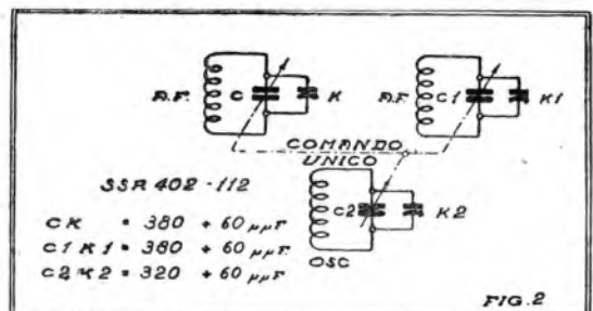
Il comando unico di una super effettuato mediante un condensatore speciale con settore per l'oscillatrice, sagomato.
