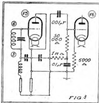
Esempio di regolatore automatico del volume. V5 è la rivelatrice funzionante come diodo. V6 è la prima di bassa frequenza.
