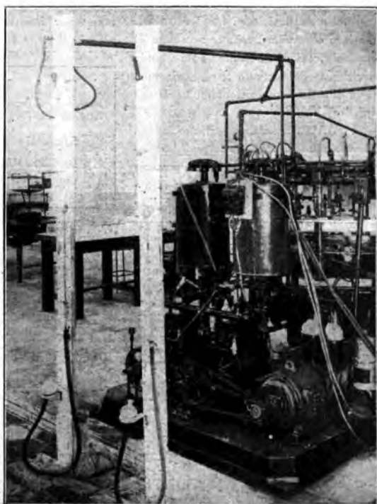
Particolare delle pompe a vuoto spinto della macchina automatica montaggio valvole.
