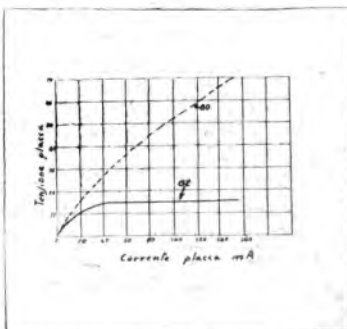
Caratteristiche del diodo rettificatore tipo 82.
