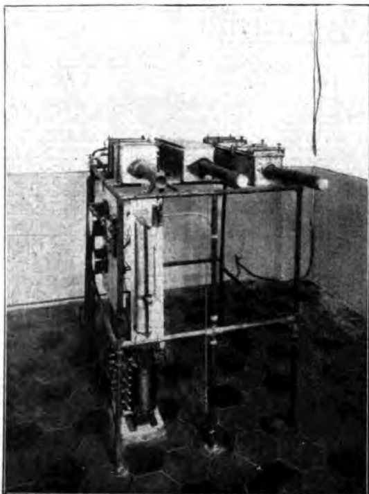
Muffole per l'idrogenazione dei filamenti.
