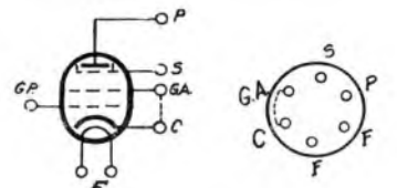
Disposizione degli elettrodi nella valvola tipo 58.
