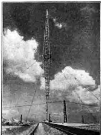
L'antenna alta 130 metri.
