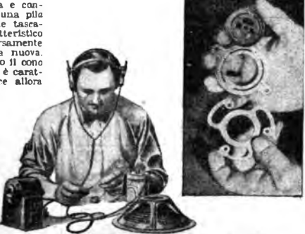
1. Con una striscia di carta si può individuare il punto di contatto tra la bobina mobile e il magnete. — 2. Con una pila a secco e una cuffia è facile riconoscere se una bobina è interrotta. — 3. Alcuni mobiletti di sistemi centranti.
