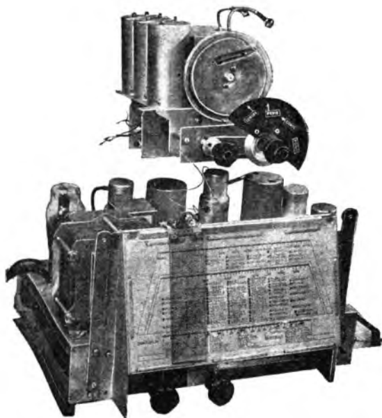
Lo chassis del TAUMANTE con il blocco di R.F. staccato
