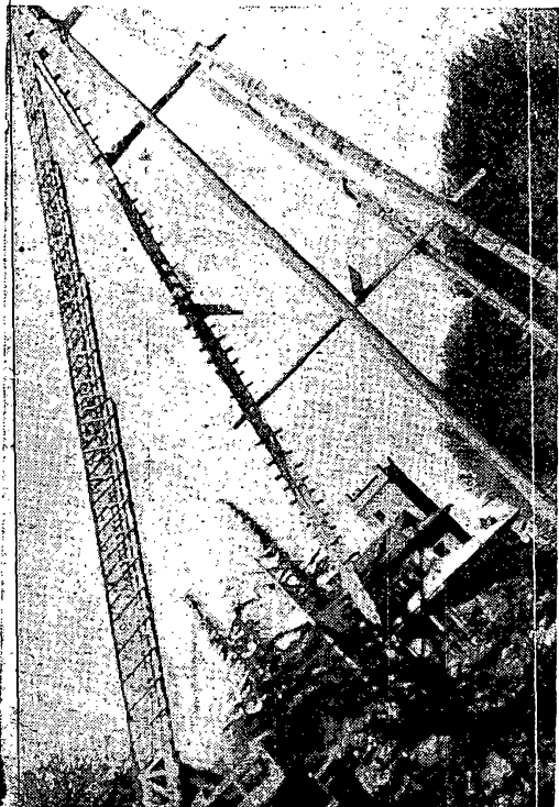
Dettaglio di sollevamento dell'antenna.
