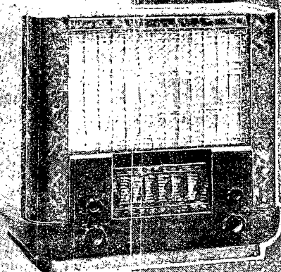
Mod. 541 M. Supereterodina 5 valvole, onde corte e medie, potenza di uscita 3 Watt indistoriti. Prezzo L. 1300 in contanti
