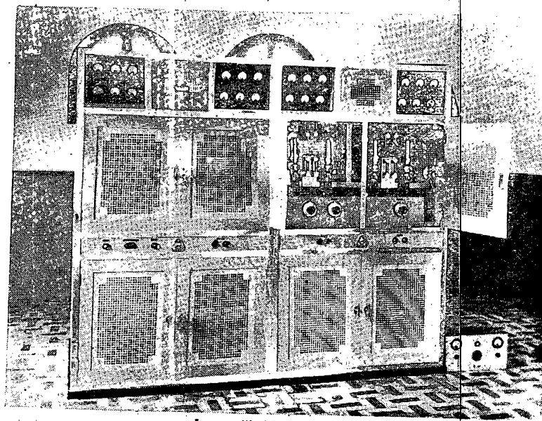
I pannelli del trasmettitore.
