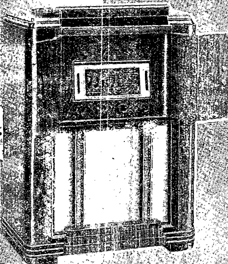
Mod. 540 G. Radiofonografo 5 valvole, onde corte, medie e lunghe, potenza di uscita Watt 4,3 indistoriti. Prezzo L. 3050 in contanti
