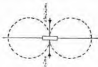
Fig. 2 - Diagramma polare di ricezione di un'antenna a telaio.
