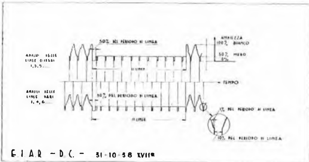
Il diagramma delle caratteristiche tecniche delle trasmissioni televisive.
