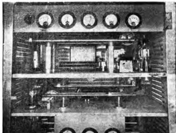
Un particolare delle stadi finali del trasmettitore M. P. della R.A.I. funzionante a Milano nel palazzo di corso Sempione (in dal 1944).
