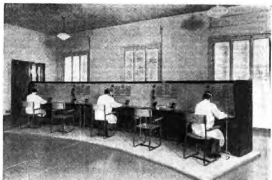
La sala controllo di Radio Torino: consente lo smistamento di cinque programmi contemporanei ed è dotata di dispositivi che evitano la possibilità di errori nelle manovre.
