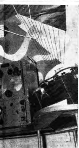
Mostra per il primo cinquantenario della Radio. originale di Marconi e di fronte ad esso un aereo in una parola, della tecnica radiofonica in questo un misuratore di campo. L'apparecchio è trasportabile nella banda di frequenza di 150 KC/s - 25 MC/s.
