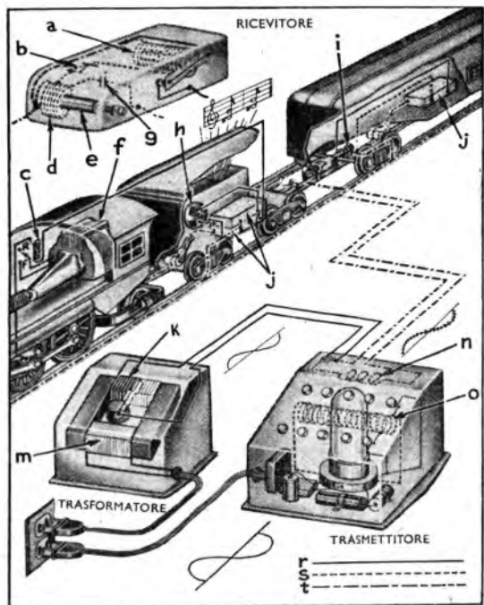
Schema dei collegamenti del modello americano Lionel
