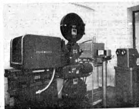
● A destra: Lo speciale apparecchio adoperato per la proiezione di film da trasmettere in televisione.
