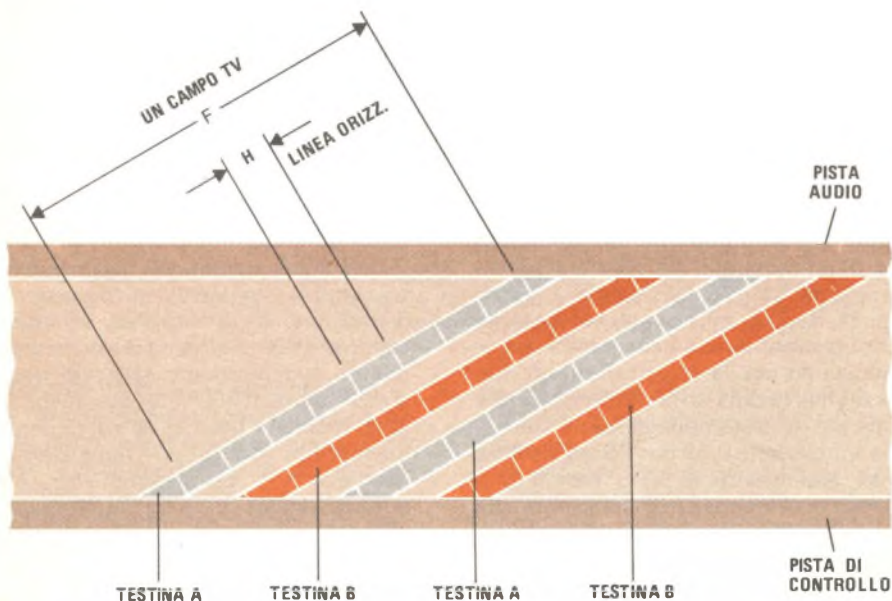
Fig. 4 - L'asse del tamburo che porta le testine è inclinato in modo che le testine scrivano su piste diagonali. La pista audio e quella di controllo vengono registrate da testine fisse.
