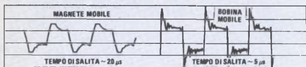
Fig. 2 - Risposte di una testina a magnete mobile (a sinistra) e di una testina a bobina mobile (a destra).
