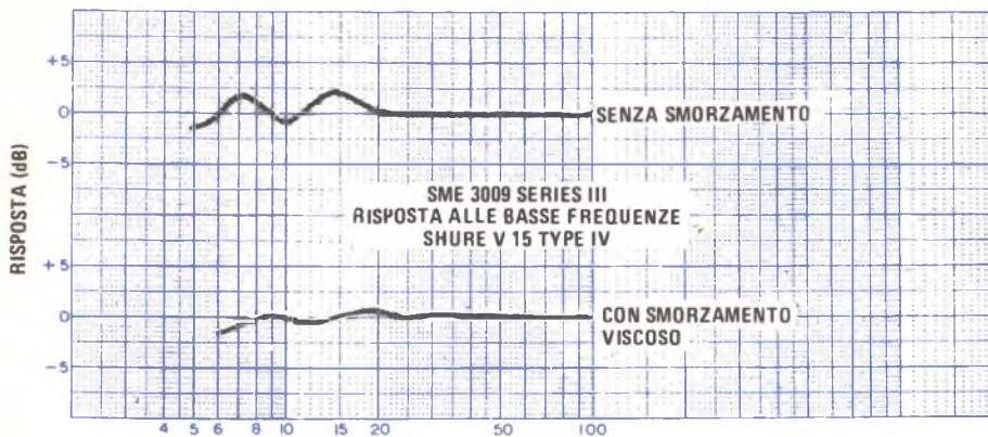
Confronto tra le risposte alle basse frequenze misurate in condizioni normali e con smorzamento viscoso.
