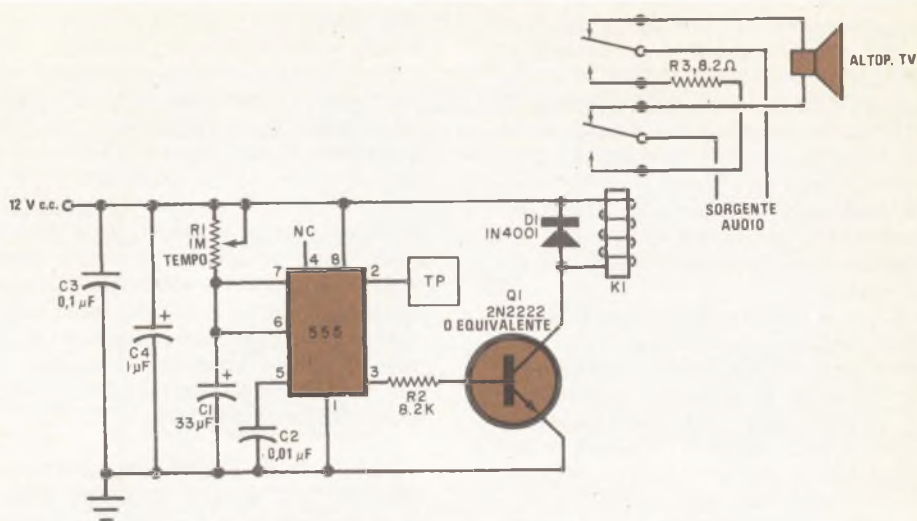
Fig. 1 - In questo circuito silenziatore per televisori viene usato l'onnipresente circuito integrato 555.
