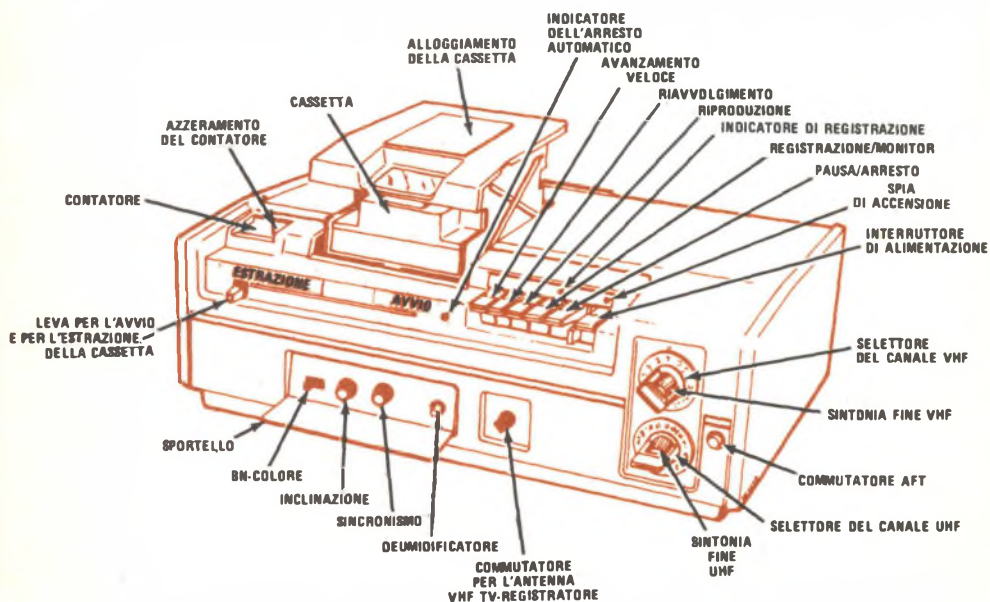
Un esempio dell'insieme dei comandi di un video registratore a cassetta (Quasar Mod. VR-1000).
