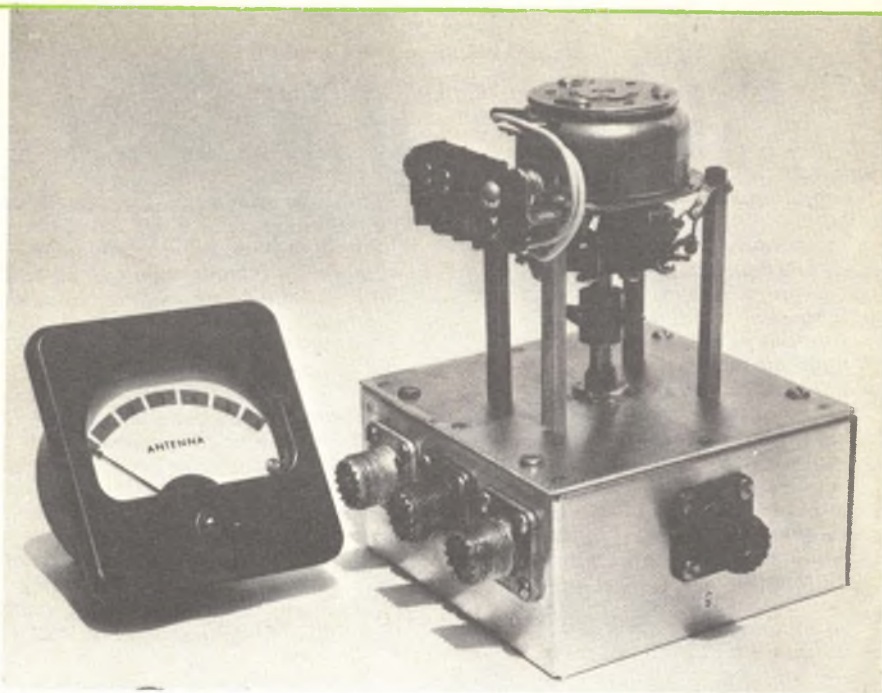
Fig. 2 - Fotografia dell'unità di commutazione a distanza e dell'indicatore dell'antenna scelta.
