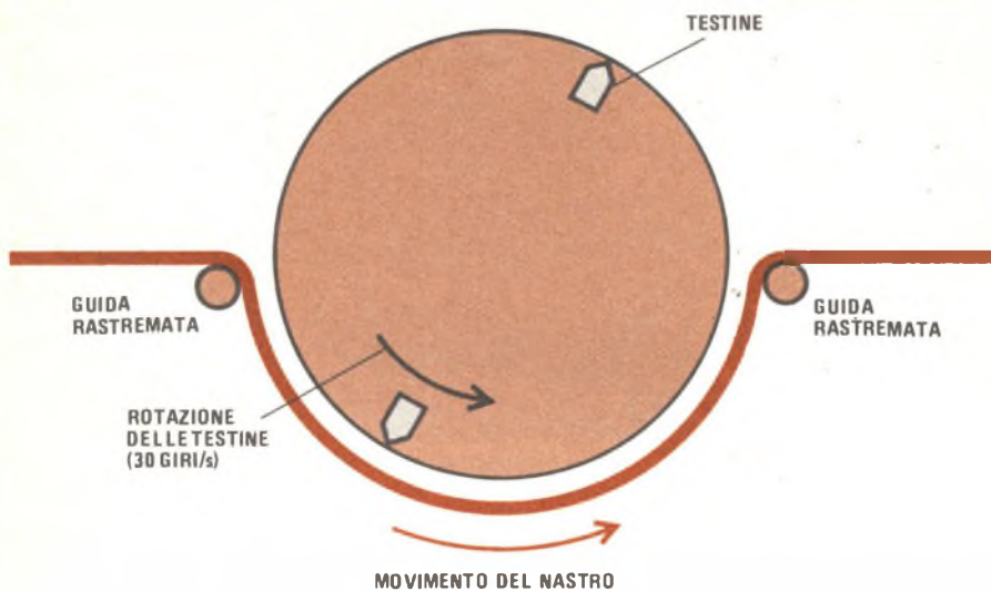
Fig. 3 - Con il nastro avvolto lungo metà della circonferenza del tamburo che porta le testine, la seconda testina inizia a registrare il secondo campo non appena la prima testina ha finito di registrare il campo precedente.
