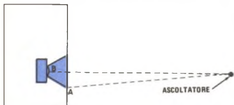
Fig. 1 - A causa della propagazione più veloce attraverso il cono, il suono generato nel punto A raggiunge l'ascoltatore prima di quello che nasce in B, punto in cui il suono di uscita dovrebbe avere origine.
