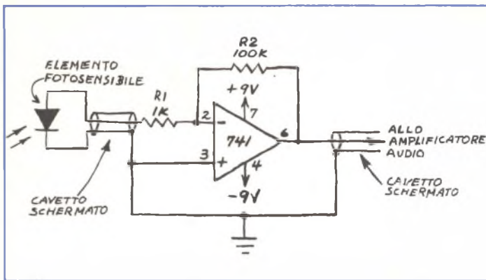
Fig. 3 - Semplice preamplificatore con amplificatore operazionale per ascoltare sorgenti di luce modulata.
