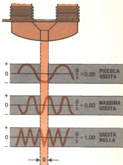
Fig. 2 - La tensione in uscita dalla testina ha un valore massimo quando la lunghezza d'onda ( \lambda ) è pari a due volte la larghezza ( g ) del traferro della testina e scende a zero quando queste due dimensioni sono uguali.
