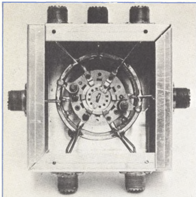
Fig. 4 - La fotografia della galletta di commutazione RF mostra due anelli di rame che vengono usati per ridurre al minimo il disadattamento delle impedenze.
