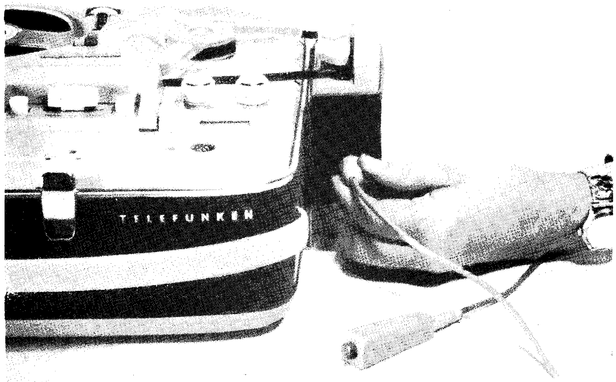
Zapojení synchronizátoru „Diachron-universal“ k magnetofonu
