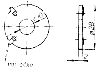
Obr. 51. Neosazené mezikruží
