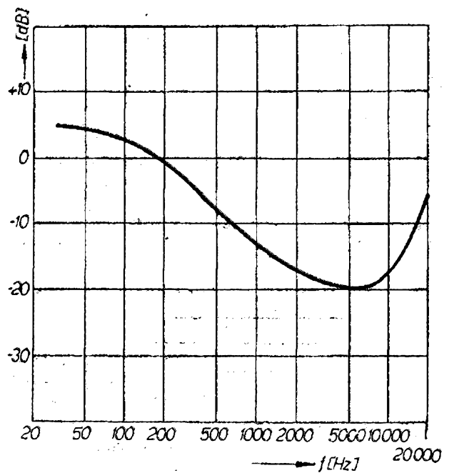
Obr. 21. Korigovaný průběh kmitočtové charakteristiky reprodukčního zesilovače
