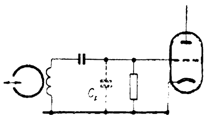
Obr. 61. Vstupní obvod reprodukčního ře- tězce elektronkového magnetofonu
