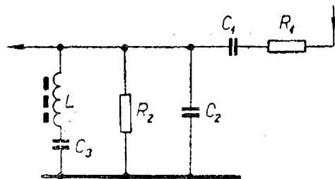
Obr. 60. Zapojení korekčního obvodu reprodukčního zesilovače
