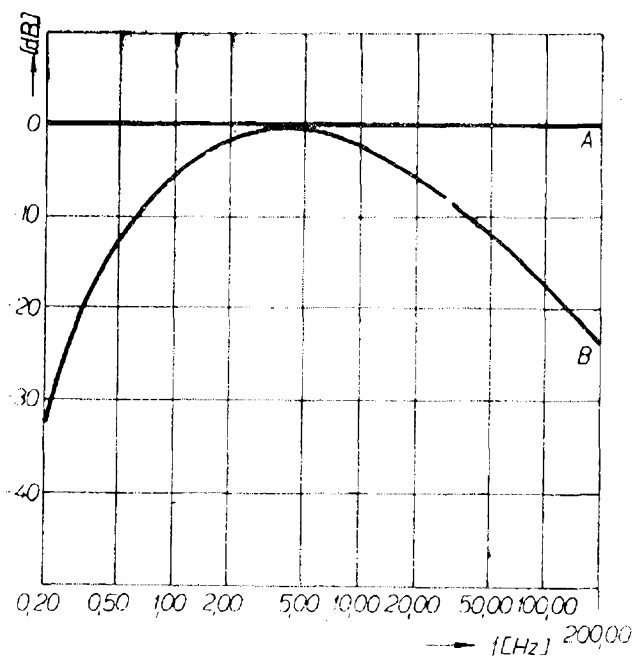
Obr. 40. Kmitočtová charakteristika filtru měřiče kolísání, pracujícího metodou závislou na vlastnostech sluchu („gehörriichtig“)
