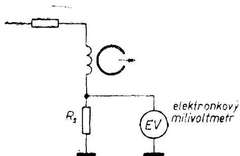
Obr. 42. Měření předmagnetizačního nebo záznamového proudu v hlavě
