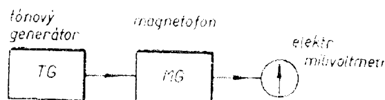
Obr. 36. Sestava přístrojů pro měření kmitočtové charakteristiky
