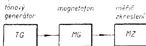
Obr. 41. Sestava přístrojů pro měření zkreslení
