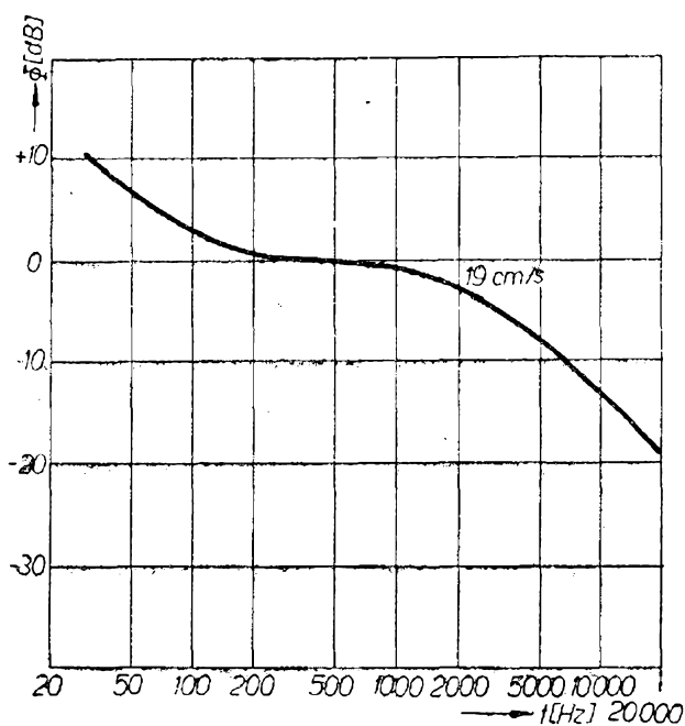
Obr. 17. Průběh magnetického toku pásku podle normy ČSN pro rychlost posuvu 19 cm/s
