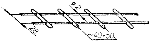
Obr. 75. Napáječ s impedancí 400 Ω pro kosočtverečnou anténu
