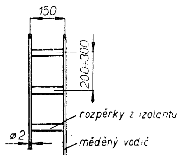
Obr. 86. Rozměry napáječe („žebříčku“) s impedancí 600 \Omega
