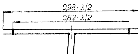
Obr. 90. Skládaný dipól z dvoulinky
