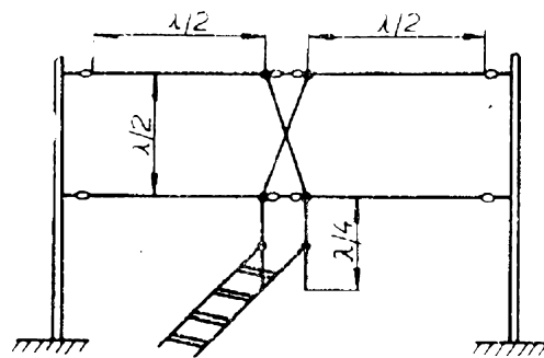
Obr. 103. Anténa typu „ležaté H“
