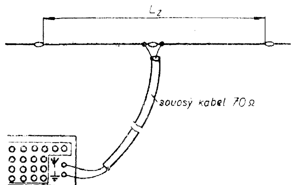
Obr. 33. Dipól pro příjem rozhlasu na KV
