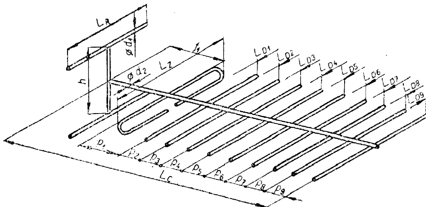
Obr. 66. Dvanáctivrvková anténa pro IV. a V. televizní pásmo
