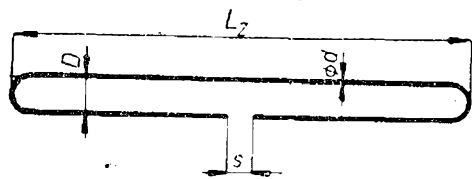
Obr. 58. Skládaný dipól
