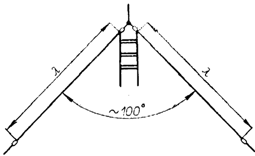
Obr. 100. Anténa typu V (pohled shora)
