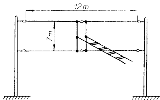
Obr. 104. Anténa „ležaté H“ pro pásma 10, 15 a 20 m
