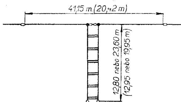
Obr. 98. Souměrná anténa typu Zeppelin
