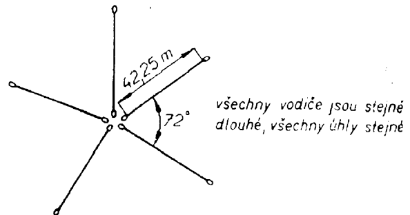
Obr. 102. Hvězdicová anténa
