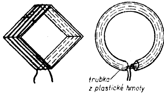
Obr. 24. Rámová anténa
