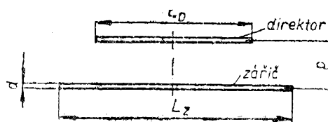
Obr. 116. Dvouprvková anténa Yagi
