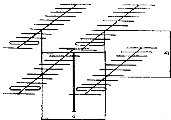
Obr. 70. Čtyřnásobná anténa
