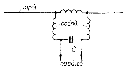
Obr. 55. Elektrické schéma bočníkového dipólu
