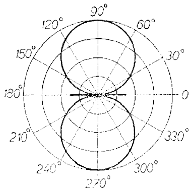
Obr. 7. Vyzářovací diagram půlvlnného dipólu
