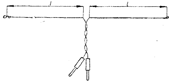
Obr. 44. Provizorní dipól
