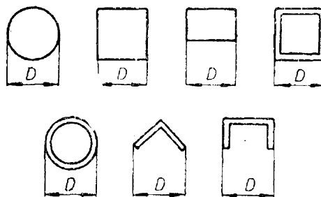
Obr. 41. Profily tyčí, použitelných pro konstrukci antén Yagi
