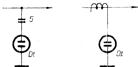
Obr. 125. Použití doutnavky k indikaci vf napětí na anténě
