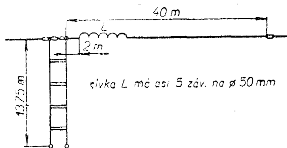
Obr. 93. Anténa DL7AB
