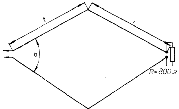
Obr. 73. Kosočtverečná anténa
