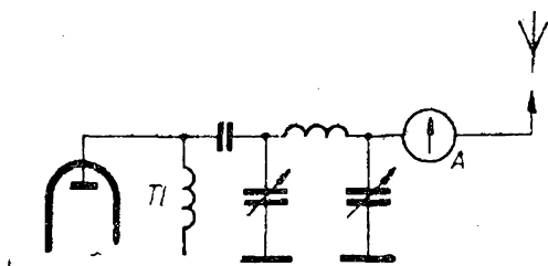
Obr. 122. Měření anténního proudu
