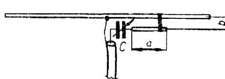
Obr. 118. Přizpůsobení antény Yagi k napájecí transformaci Gamma
