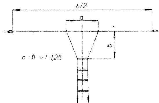
Obr. 19. Transformace Delta
