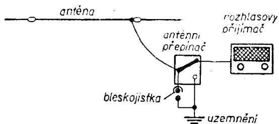
Obr. 32. Připojení bleskojistky a anténního přepínače
