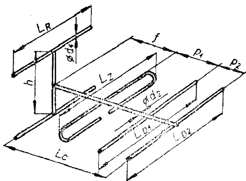
Obr. 65. Pětivrvková anténa pro IV. a V. televizní pásmo
