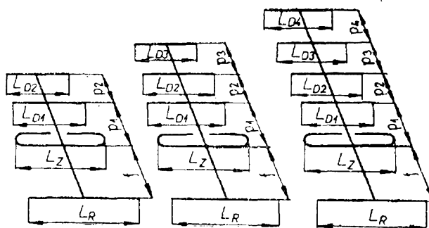
Obr. 40. Čtyř-, pěti- a šestiprvková anténa Yagi
