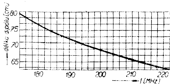
Obr. 52. Délka skládaného dipólu pro kmitočty 180 až 220 MHz
