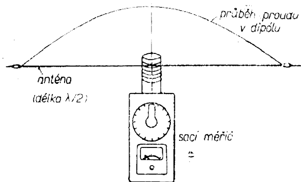
Obr. 127. Měření rezonančního kmitočtu antény sacím měřičem
