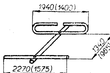
Obr. 38. Dvouprvková anténa Yagi
